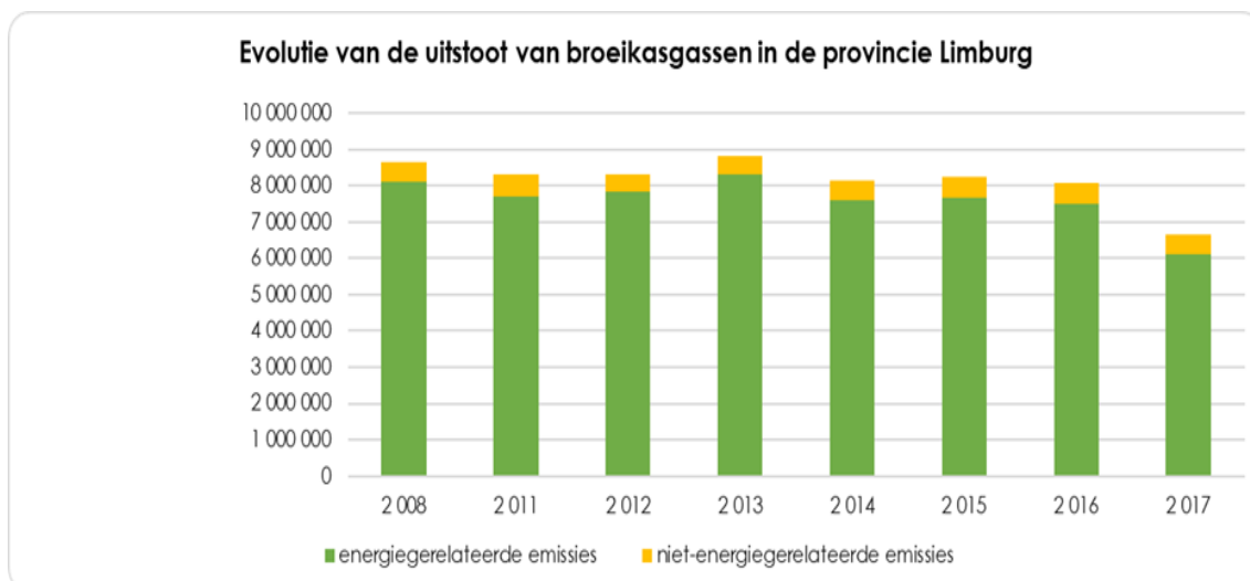
Figuur 6-4 Evolutie uitstoot broeikasgassen (in ton CO 2eq ) in Limburg voor de periode 2008 – 2017 (bron: 'Emissierapport 2015-2016-2017' (Zero Emission Solutions, 2020)).
