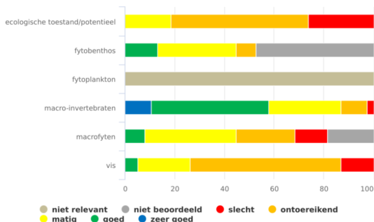
Figuur 6-13 Ecologische toestand/potentieel (2013 – 2018) Lokale waterlopen Maasbekken
