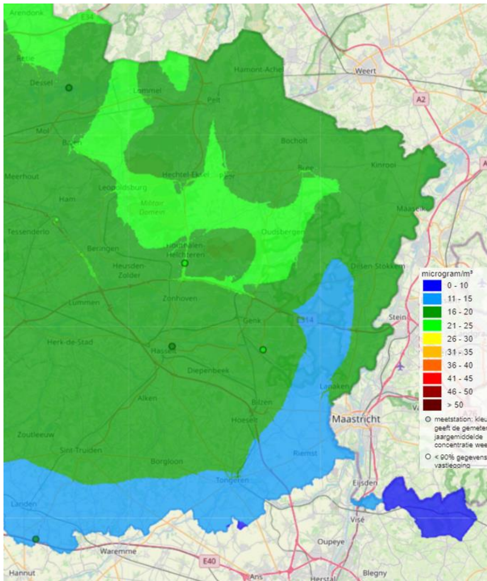
Figuur 6-50 Jaargemiddelde PM_{10} concentratie in 2019 voor de provincie Limburg (bron: VMM)
