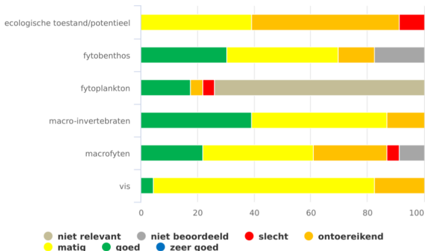
Figuur 6-9 Ecologische toestand/potentieel (2013 – 2018) Vlaamse waterlopen Demerbekken
