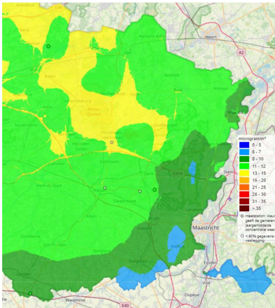
Figuur 6-51 Jaargemiddelde PM 2,5 concentratie in 2019 voor de provincie Limburg (bron: VMM)
