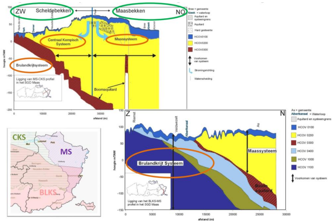
Figuur 6-8 Plangebied Limburg – grondwatersystemen
