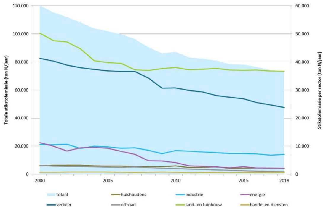
Figuur 6-62 Stikstofemissies per sector tussen 2000-2018
